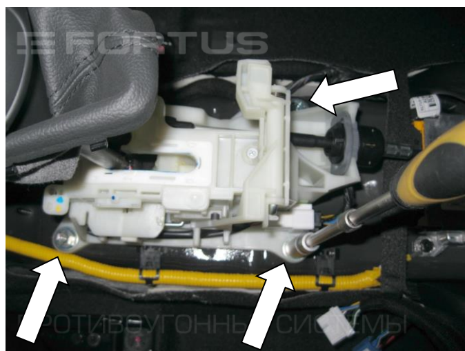
10. Открутите три болта крепления селектора
