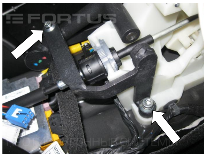
12. Установите кронштейн (поз. 3), закрепив болтами (поз. 6, 9) с шайбами (поз. 10, 11)
