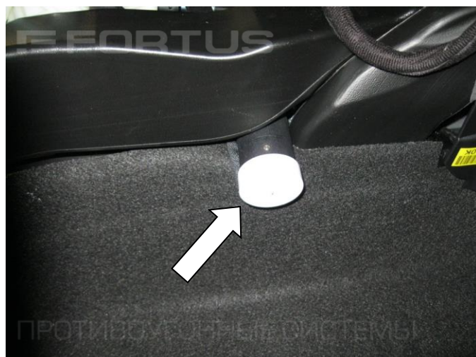
14. Установите шаблон SCH7 на корпус замка
