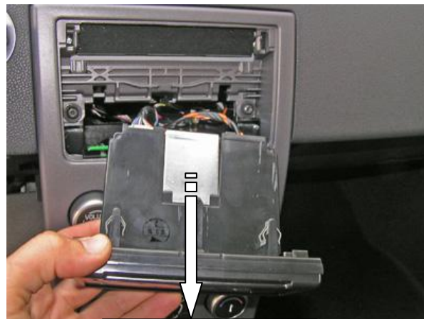
Снять магнитолу
